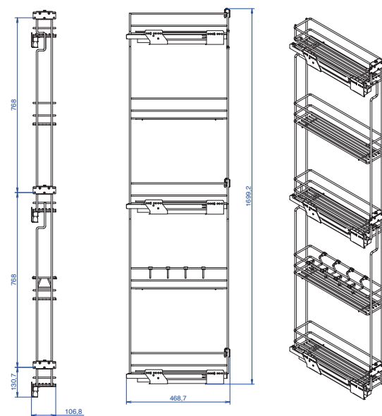
Estraibile laterale 5 piani 5 shelves pull-out unit
